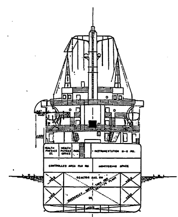
付図-1 一般配置図 (1/2)
